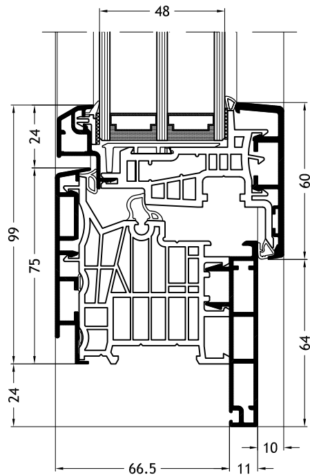
Aro em forma de L D1Z com folha Classic-line A27
