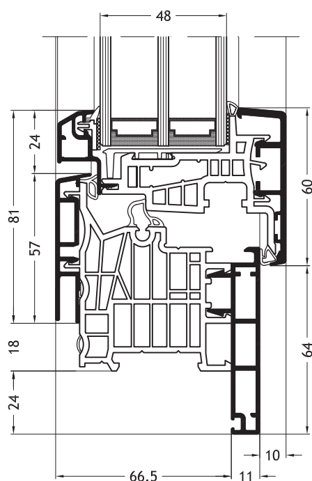
Aro em forma de L D1V com folha Classic-line A27
