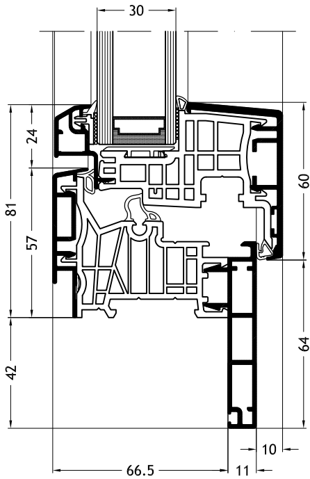
Aro em forma de Z D2Y com folha Classic-line A26
