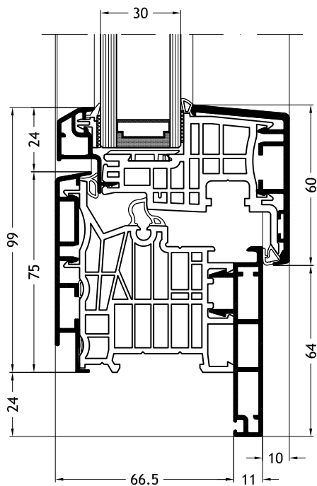
Aro em forma de L D1Z com folha Classic-line A26
