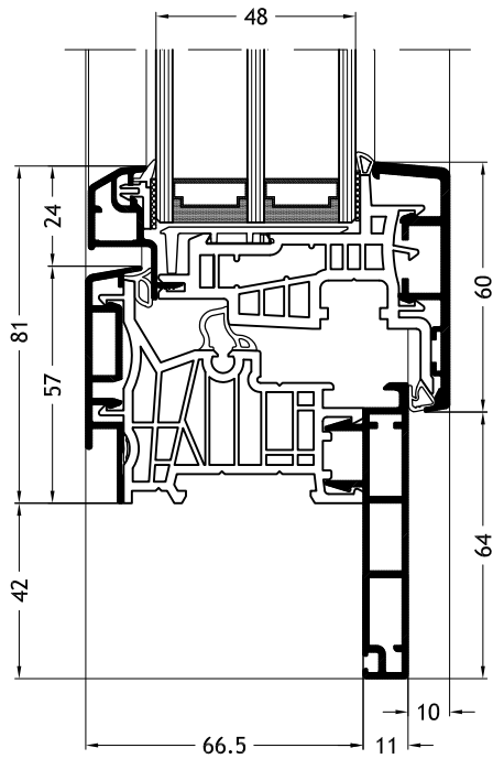
Aro em forma de Z D2Y com folha Classic-line A27
