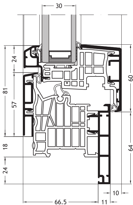
Aro em forma de L D1V com folha Classic-line A26
